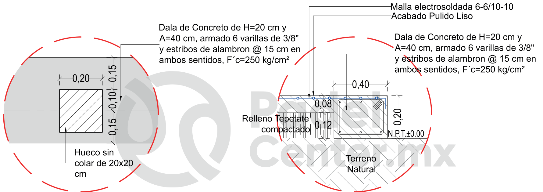
DET 01 DETALLE CONSTRUCTIVO
